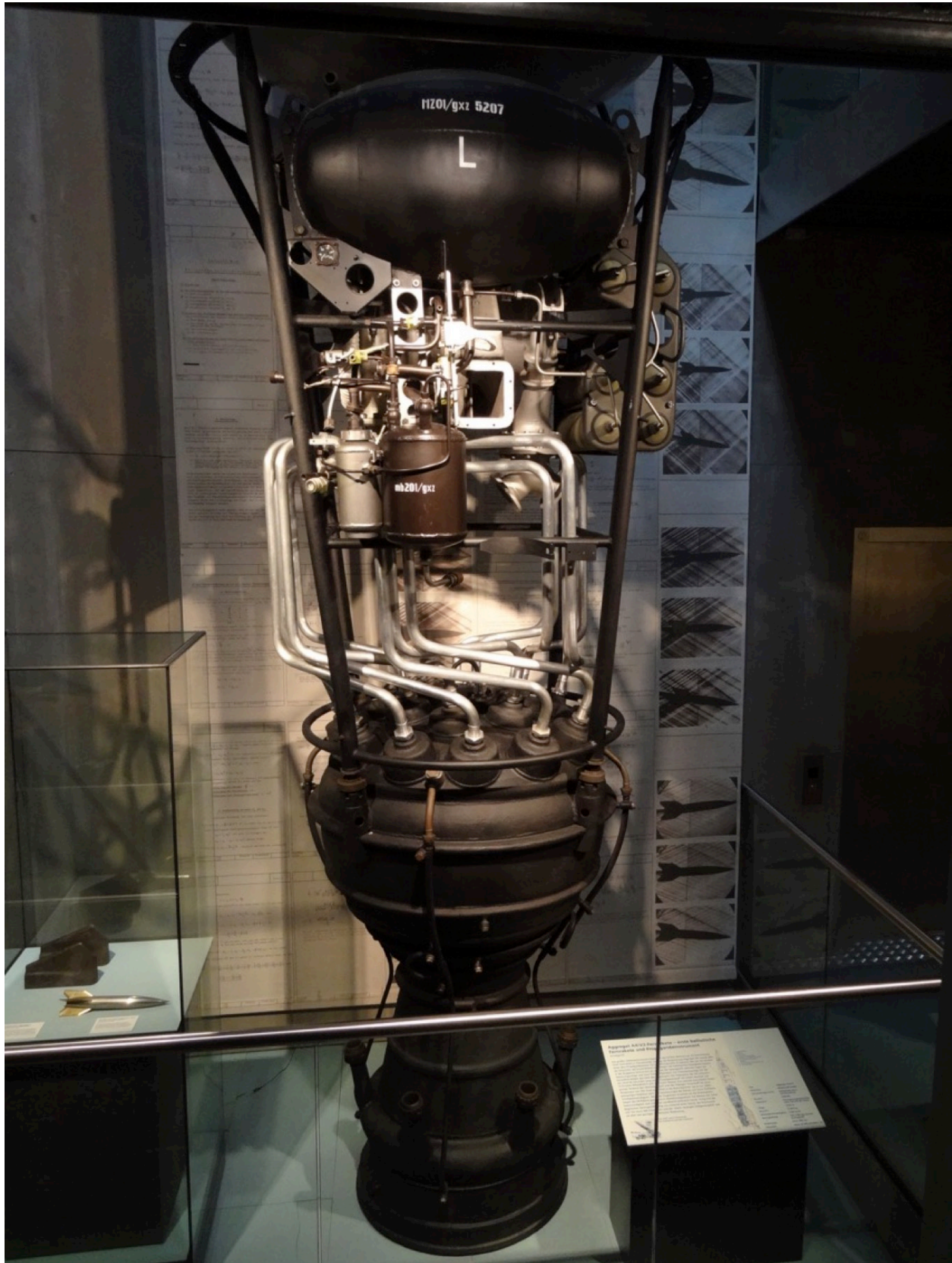
Figure E.46: A-4 rocket engine in Deutsches Technikmuseum Berlin.
