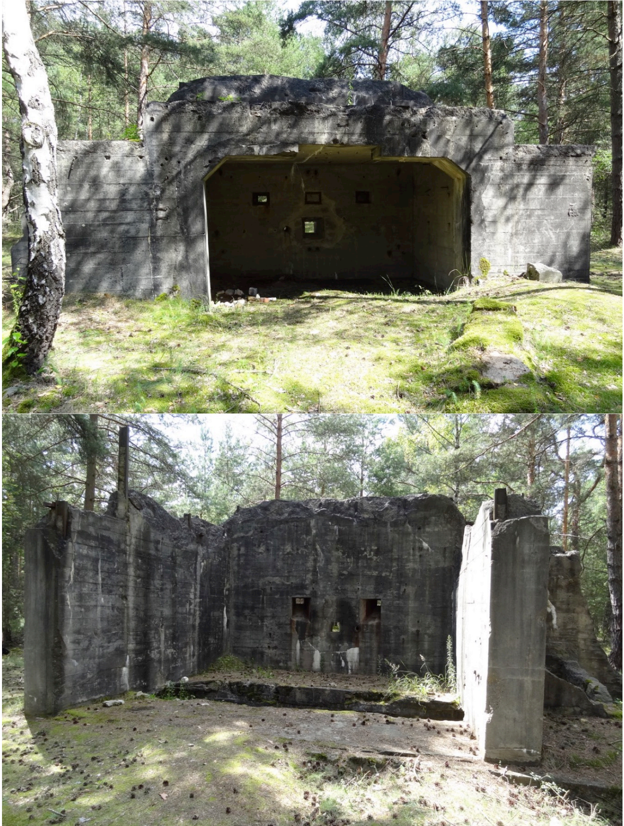
Figure E.39: Historisch-Technisches Museum Versuchsstelle Kummersdorf: A-3 rocket test stand and control bunker.
