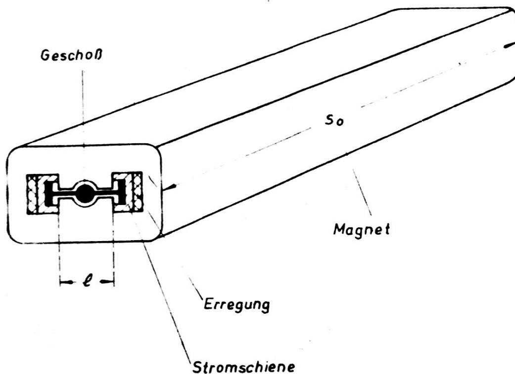
Linearmotor Bild 1
